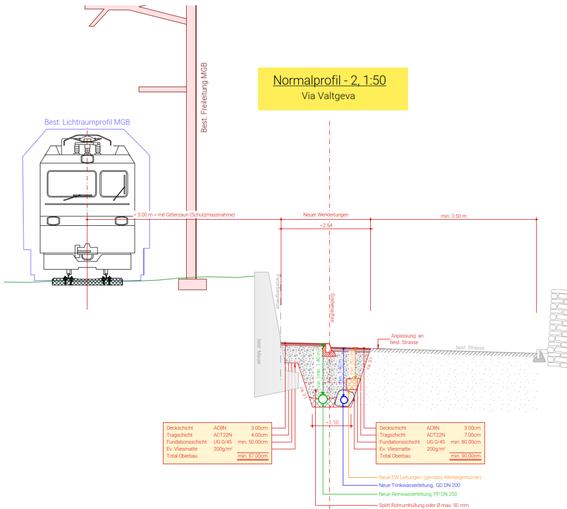
Profil 1:50
