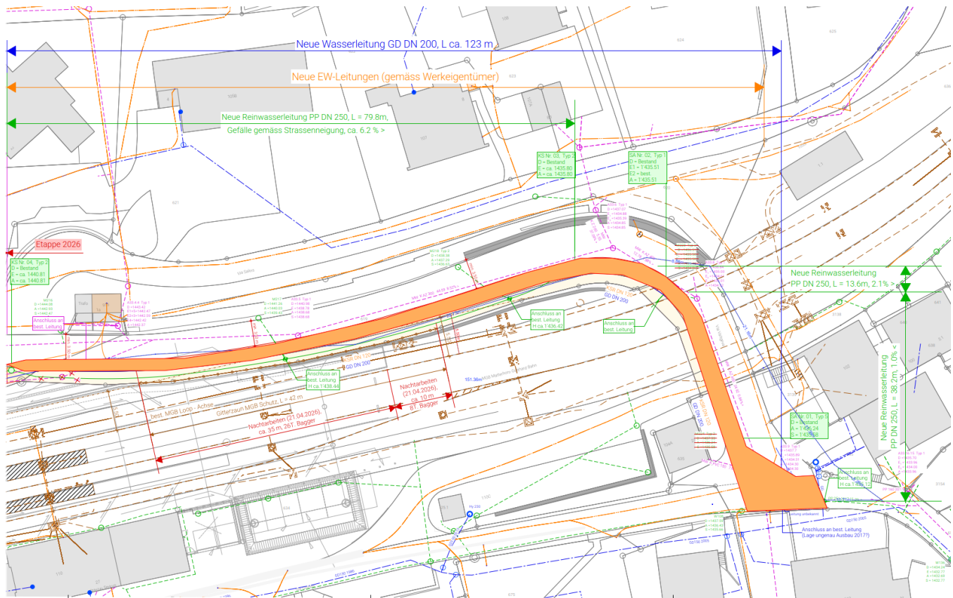
Plan da situaziun e canalisaziun 1:200
