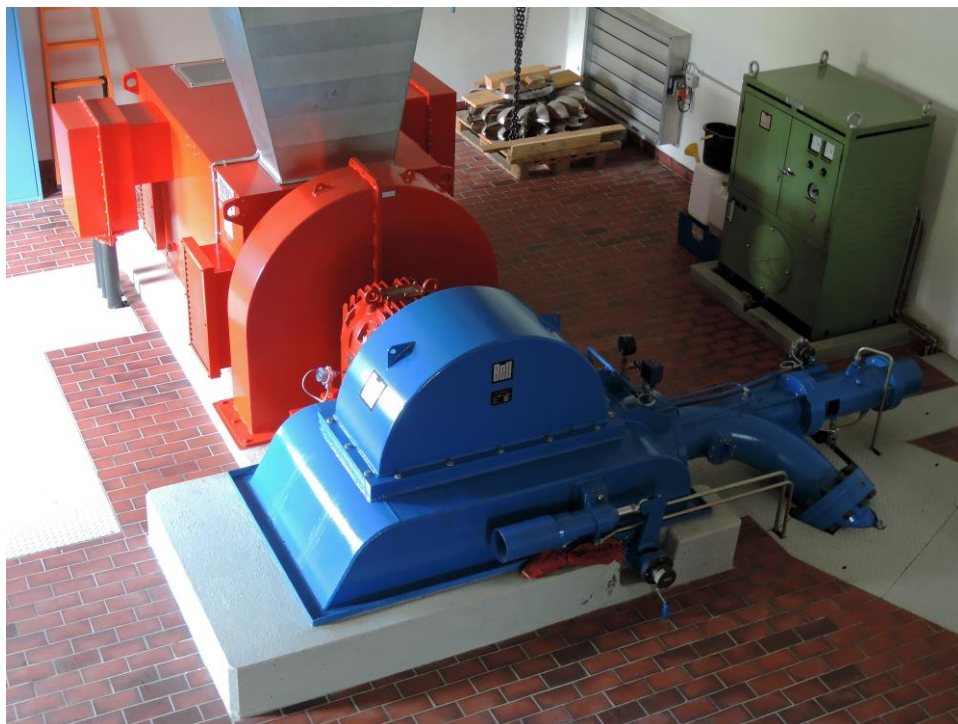
foto 7: ella centrala la turbina existenta cun generatur
